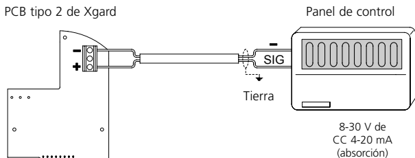
Diagrama 7: conexiones eléctricas de Xgard tipo 2
