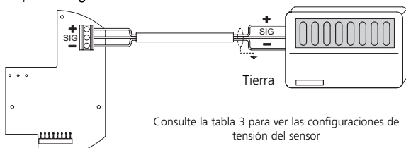
Diagrama 9: conexiones eléctricas tipo 3 de Xgard
