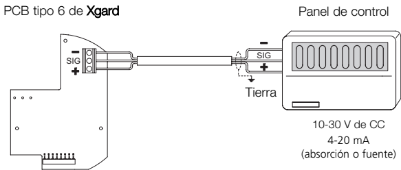
Diagrama 15: conexiones eléctricas del tipo 6 de Xgard
