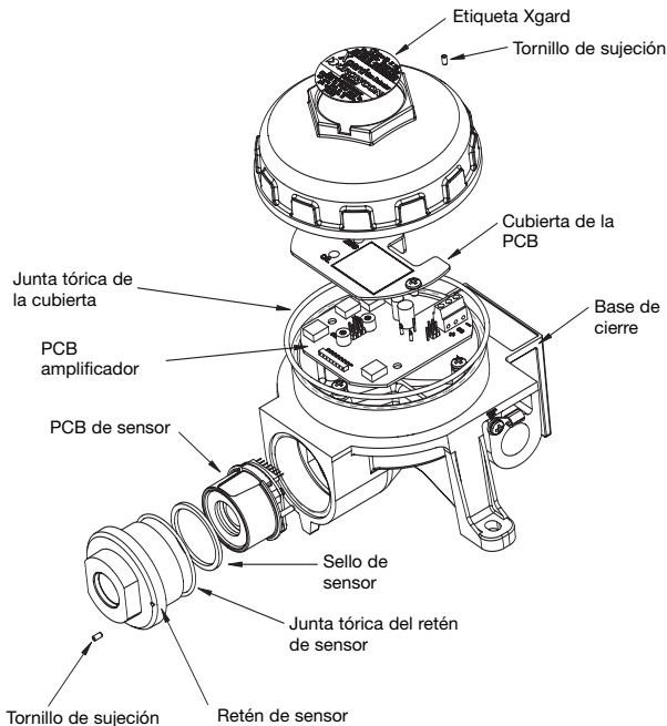
Diagrama 3: vista despiezada de Xgard (donde aplicable, los números de la parte se muestran en paréntesis). For part numbers not shown, see Spares and Accessories on page 59)
