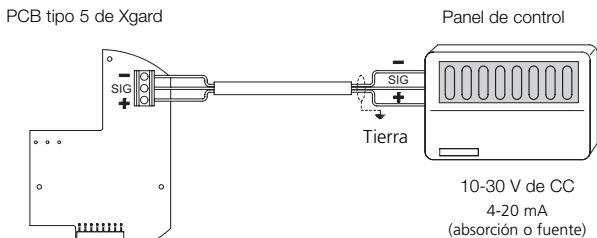
Diagrama 13: conexiones eléctricas tipo 5 de Xgard
